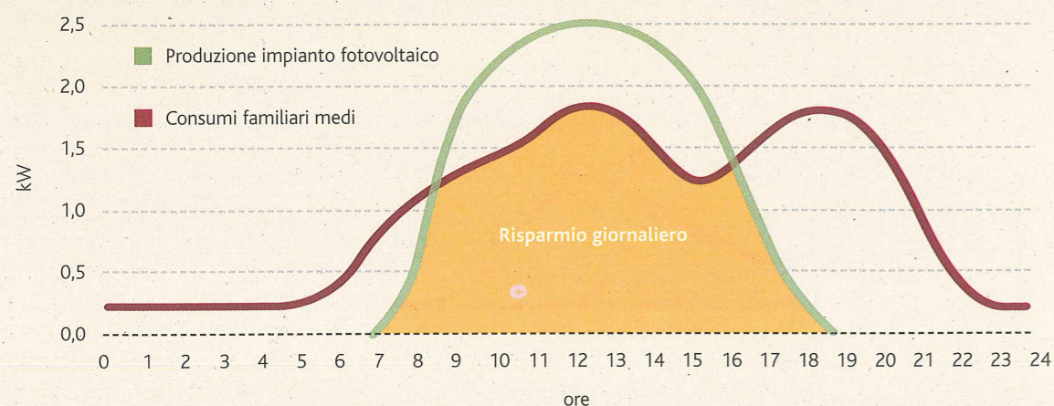
Grafico indicativo di produzione, consumi e risparmio giornaliero (impianto da 3 kWp)
